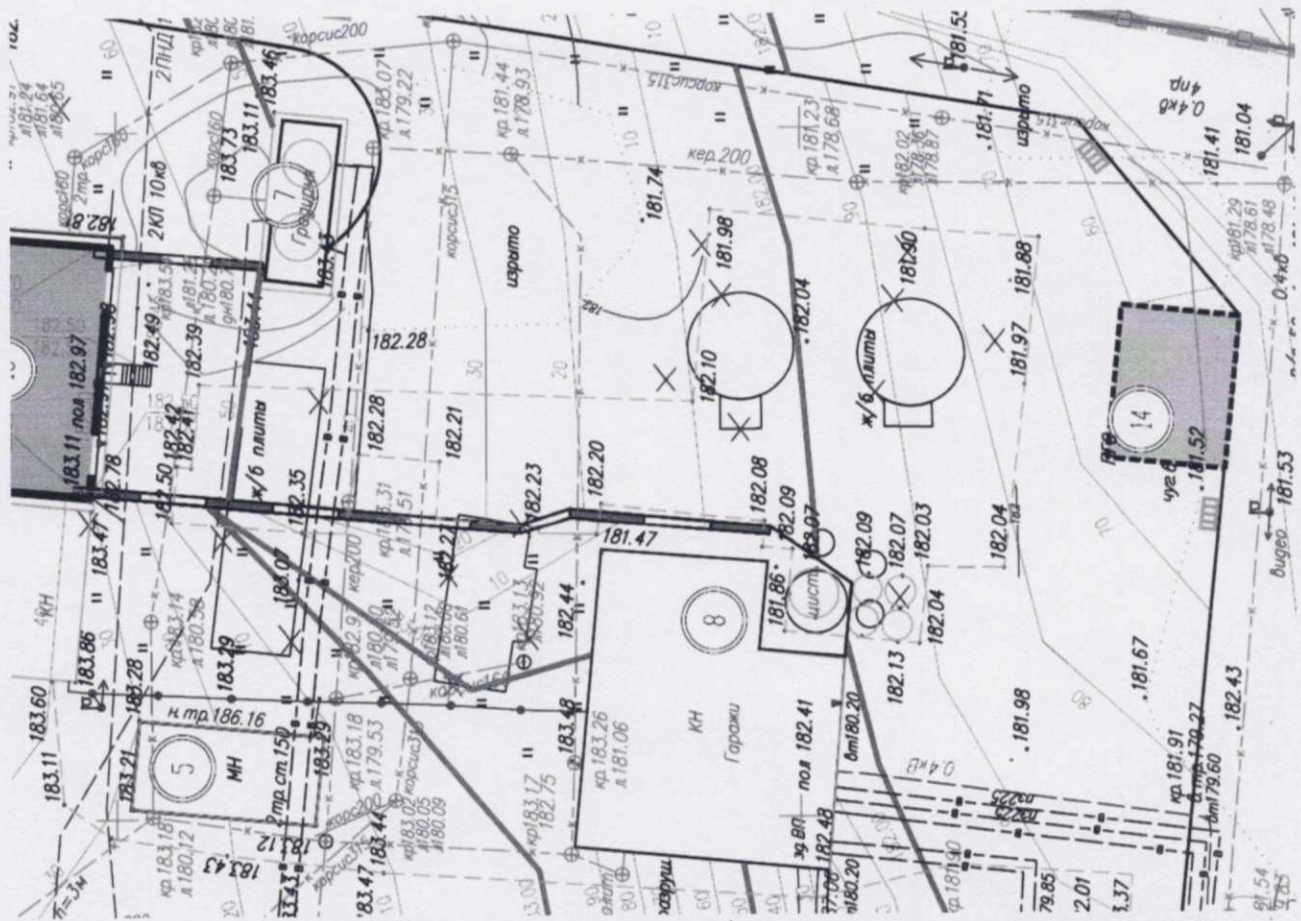
Рис.2 План организации рельефа на участке перед складом упаковки.
