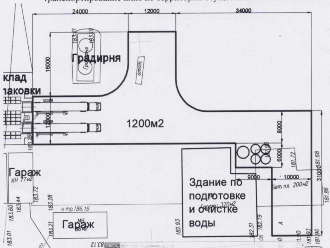
Рис.1 План траектории участка выполняемой дороги перед складом упаковки.
